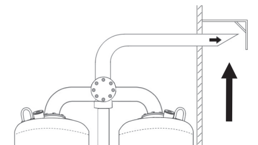
Wetterschutz bei seitlicher Verlegung der Leitung
