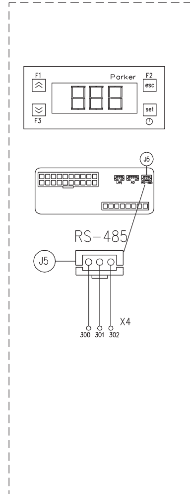
RS-485 - OPTION OPZIONE - RS485
